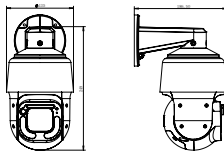
图2-1 结构尺寸示意图
