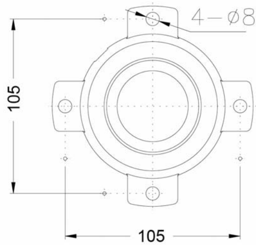
Pendant mount
