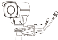
图3-1 设备安装示意图
