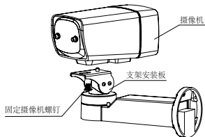
图2-1 摄像机与旋转支架连接说明
