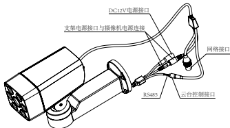
图1-2 外接线缆示意图
