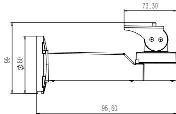
图1-3 结构尺寸示意图
