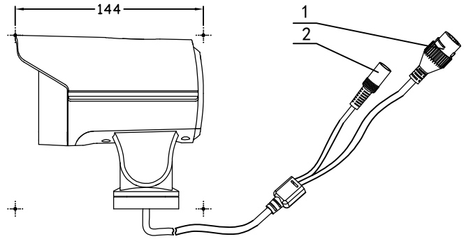
图 1-1 外接线缆示意图
