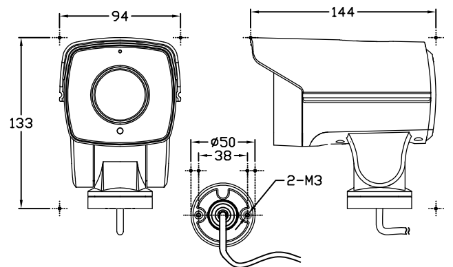
图 1-1 结构尺寸示意图
