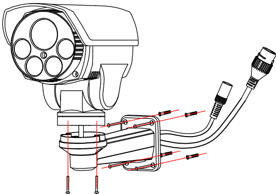
图 1-1 设备安装示意图
